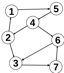
Grafo orientato
