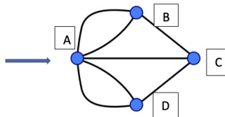
Il grafo dei sette ponti
