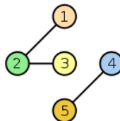
Grafo con 2 comp. connesse
