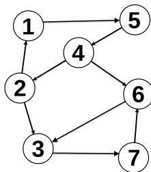
B: Grafo non Hamiltoniano
