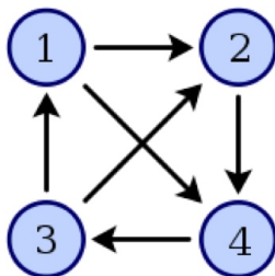
Torneo con quattro vertici
