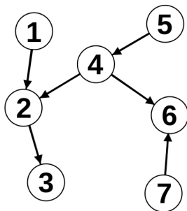
Grafo orientato debolmente connesso
