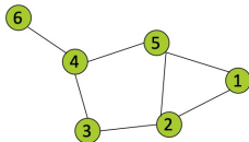
Grafo non orientato
