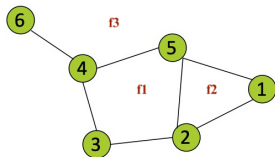
Grafo con 3 facce
