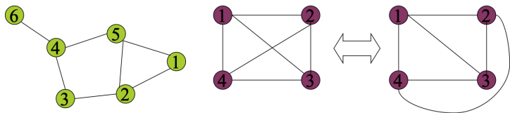
Esempi di grafi planari
