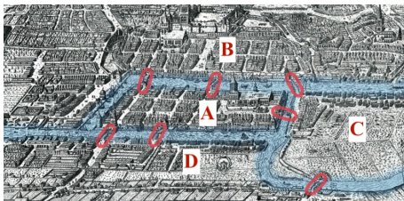
I sette ponti di Königsberg nel 1736
