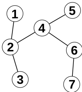
Grafo aciclico
