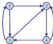
Grafo orientato
