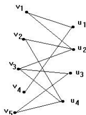
Grafo bipartito con 9 vertici
