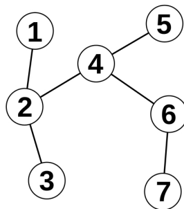
Grafo sottostante connesso
