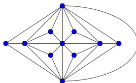
Grafo massimale con 11 vertici
