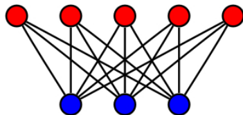
Grafo bipartito completo: K_{5,3}
