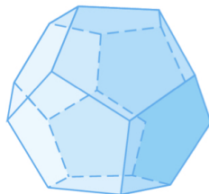
Dodecaedro
