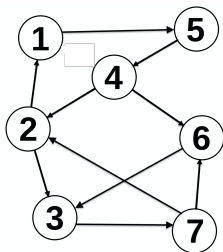
A: Grafo Hamiltoniano
