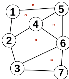
Grafo con 5 facce
