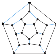
Dodecaedro schiacciato su una faccia
