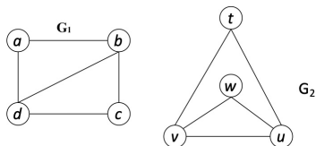
Grafi isomorfi
