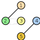
Grafo con 3 comp. connesse
