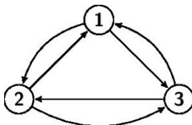
Digrafo completo con 3 vertici
