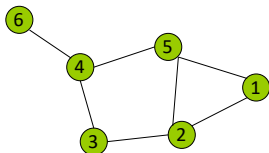
Grafo non orientato
