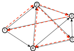
Circuito diretto: 1, 2, 5, 4, 2, 3, 1
