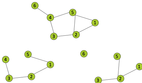
Grafo non orientato e due possibili sottografi
