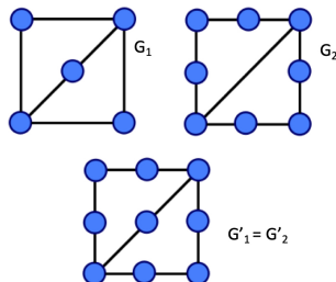
Grafi omeomorfi: Esempio
