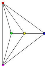
Grafo massimale con 5 vertici
