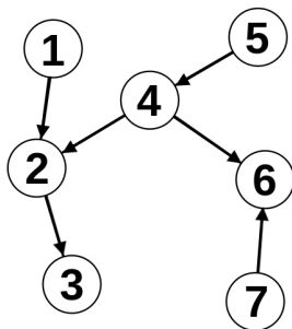
Digrafo Aciclico
