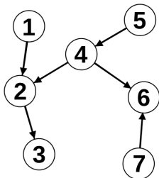
Grafo orientato
