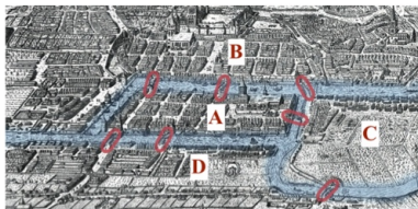
Il grafo dei sette ponti
