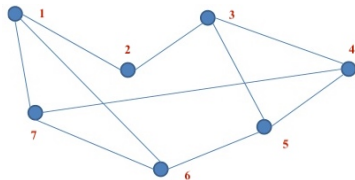
Grafo non orientato
