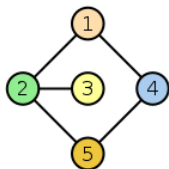
Grafo con 1 comp. connessa
