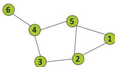
Grafo non orientato
