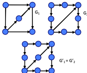
Grafi orientati omeomorfi: Esempio
